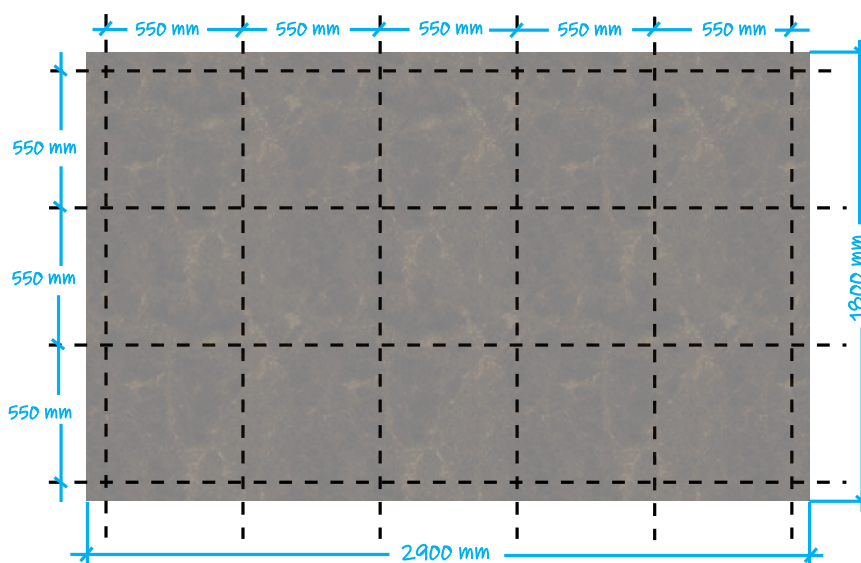
Figura 8 - Simulação de corte de chapa em ladrilhos 55 x 55 cm (22,40 m de corte).
